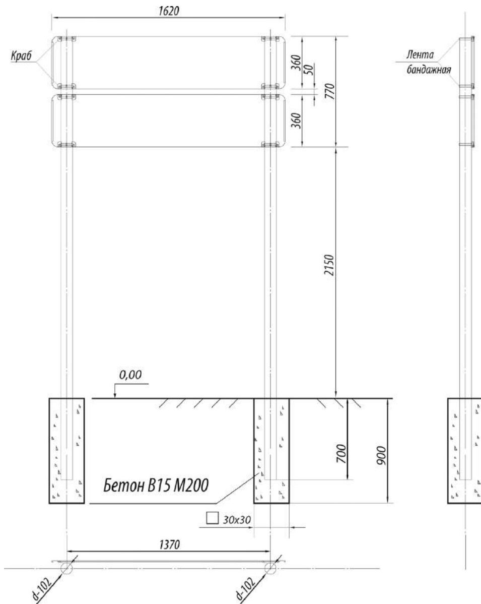
Рис.4. Конструкция туристского указателя с двумя ярусами
