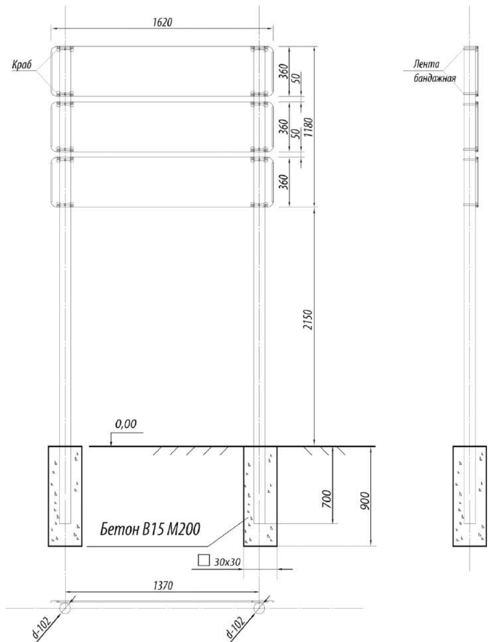
Рис.5. Конструкция туристского указателя с тремя ярусами
