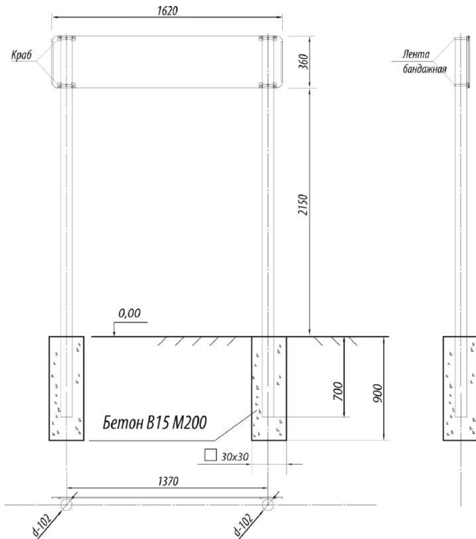
Рис.3. Конструкция туристского указателя
