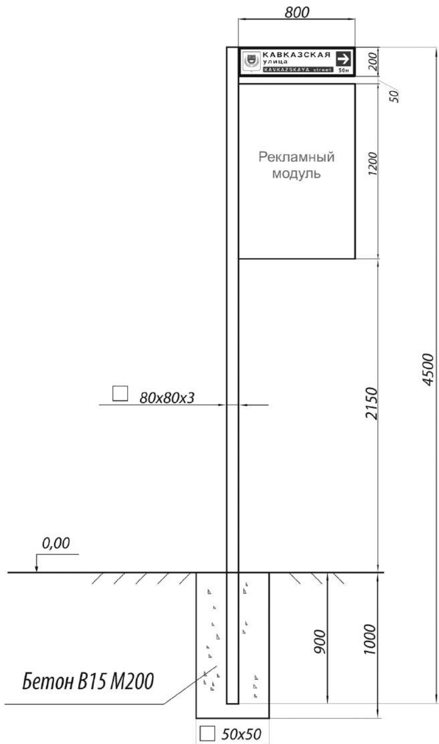
Рис. 11. Конструкция информационного указателя индивидуального проектирования с рекламным модулем
