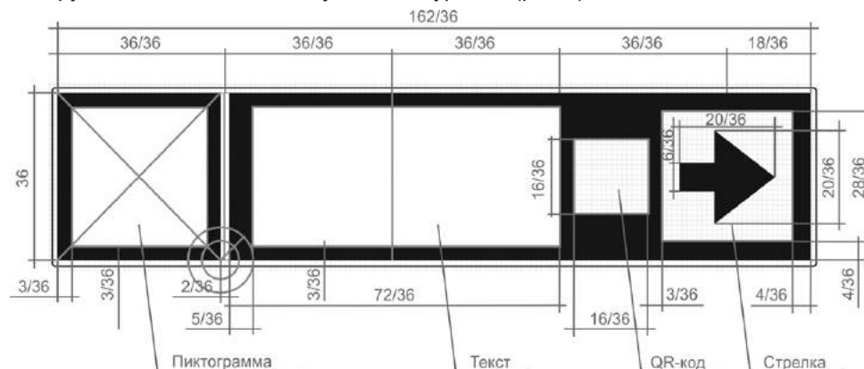
Рис. 1. Указатель туристский
