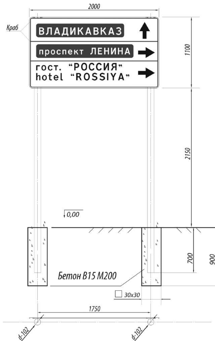
Рис. 12. Указатель направления
