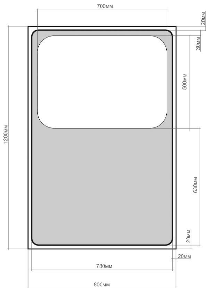
Рис.7. Информационный указатель
