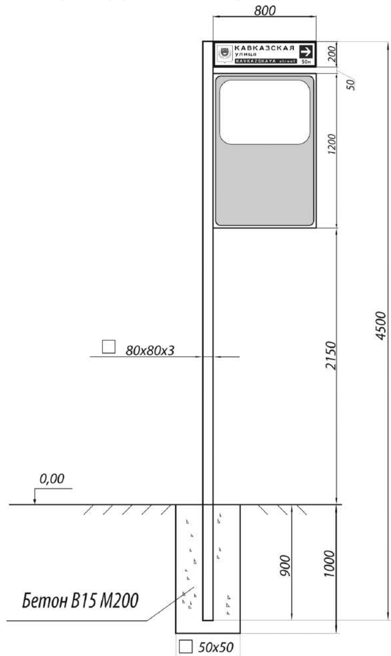
Рис.8. Конструкция информационного указателя индивидуального проектирования
