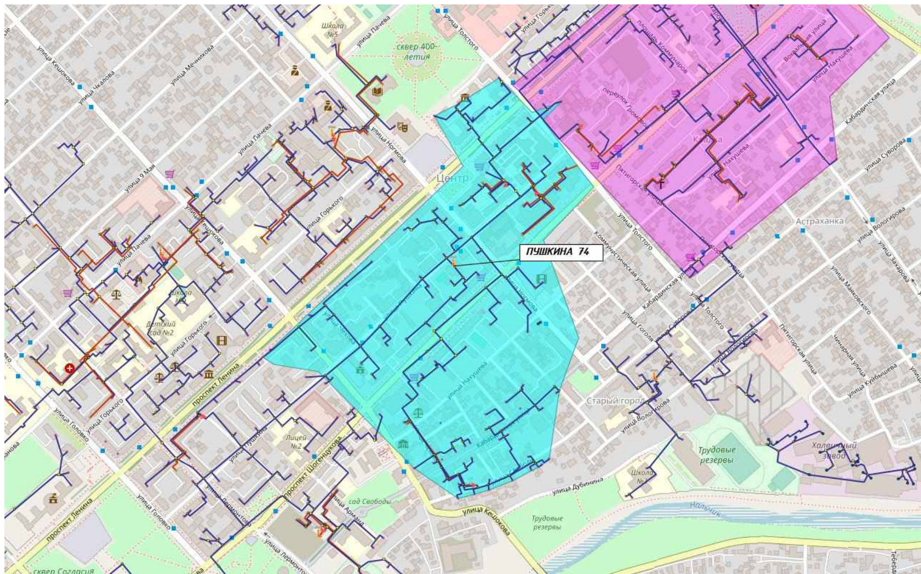
Рисунок 2.3. Существующая зона действия котельной «Пушкина»
