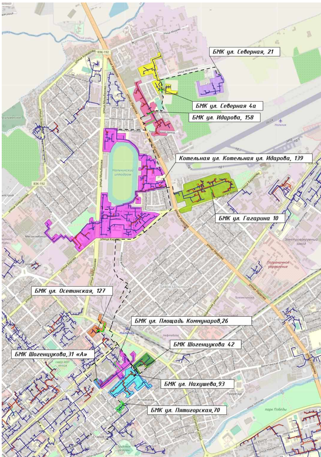
Рисунок 2.7. Зона действия перспективных котельных в рамках реализации мероприятий по децентрализации котельной «Юго-Западная»
