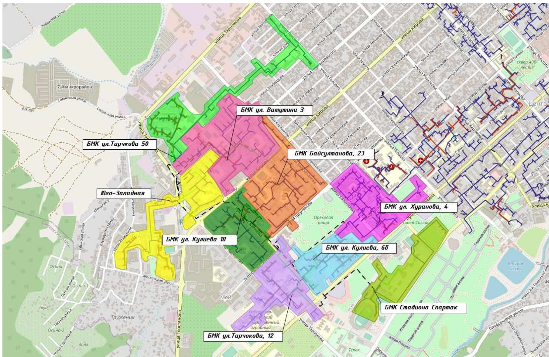
Рисунок 2.6. Зоны действия перспективных котельных в рамках децентрализации котельной «Юго-Западная»
