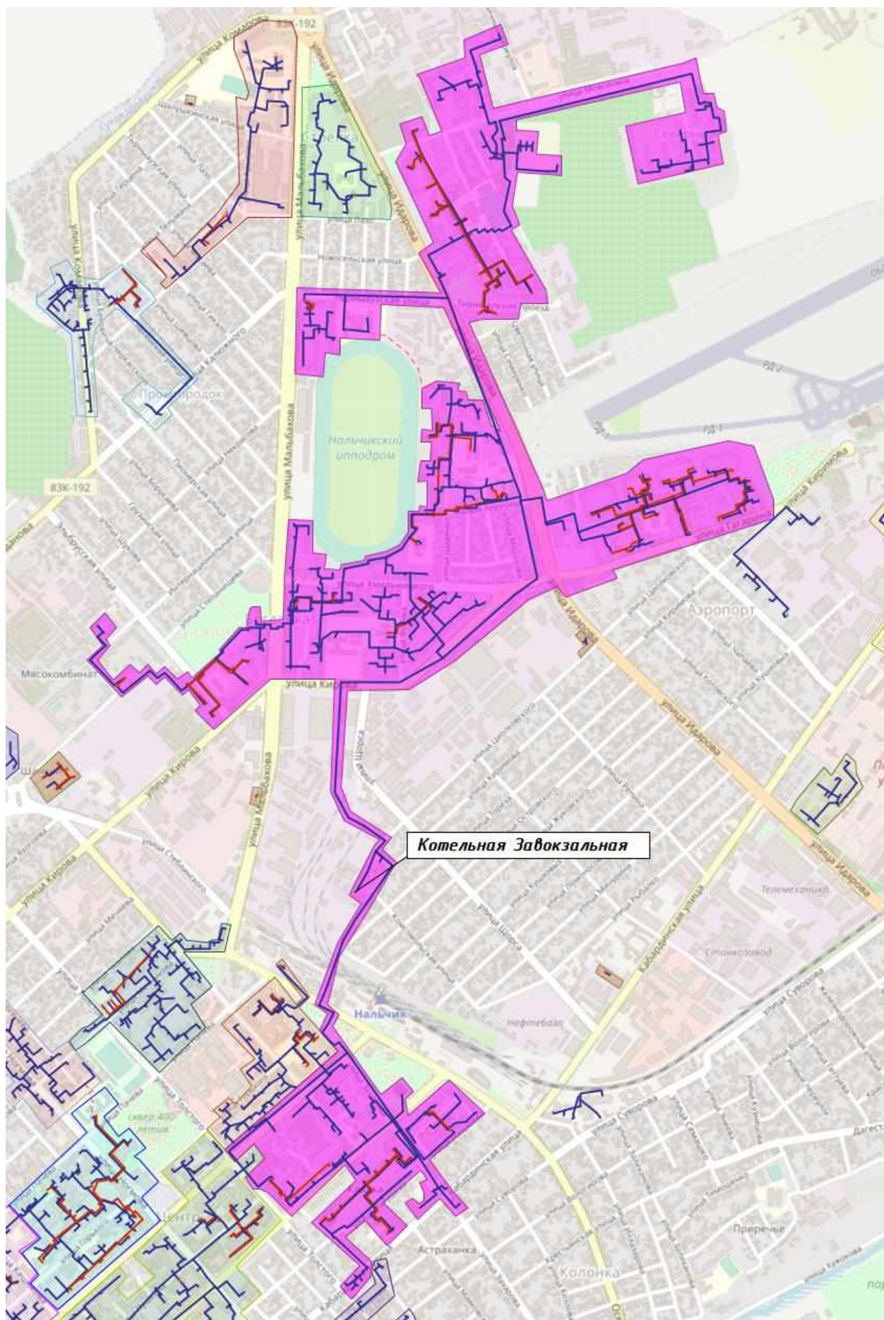
Рисунок 2.2. Существующая зона действия котельной «9 Января» («Завокзальная»)
