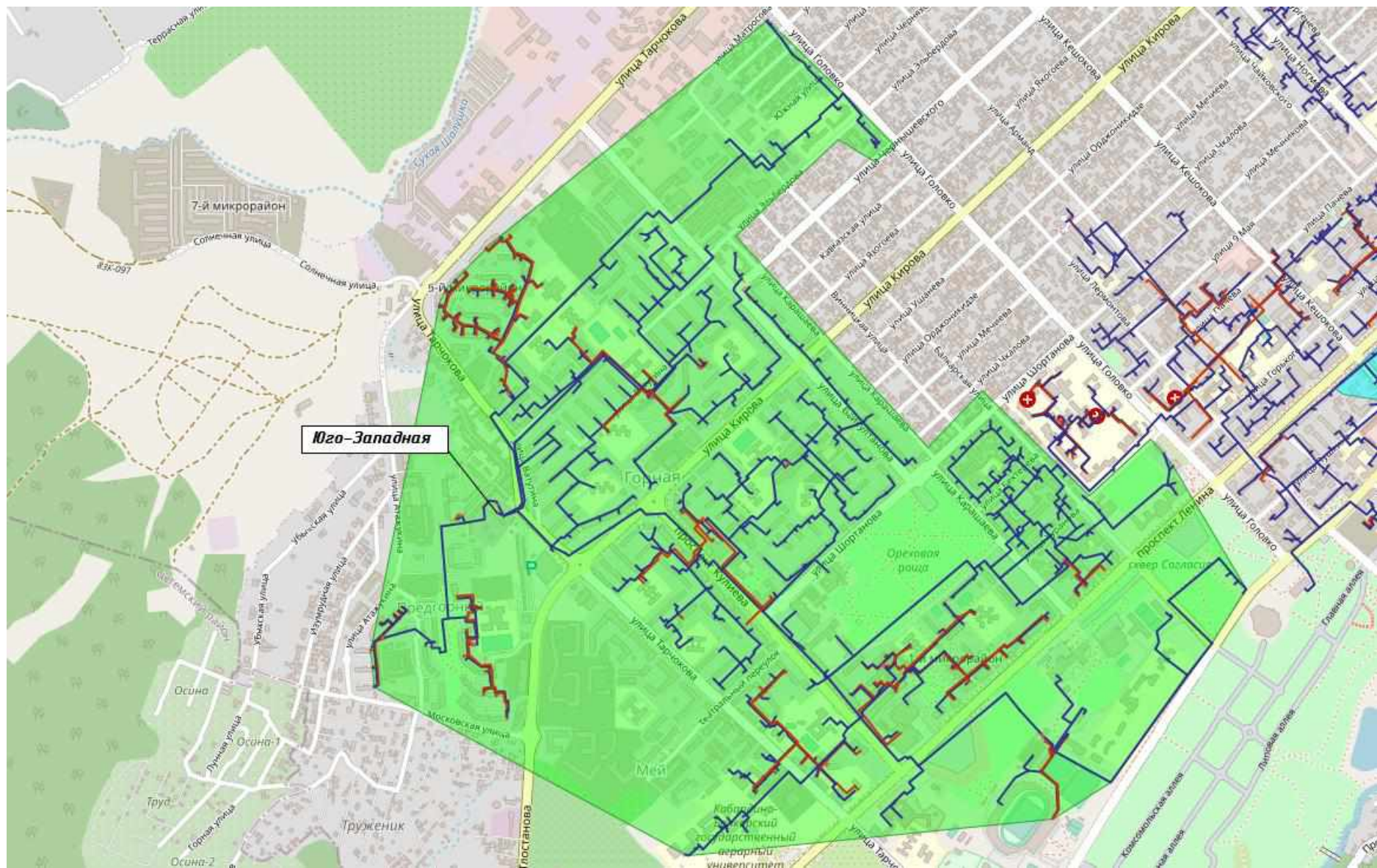
Рисунок 2.1. Существующая зона действия котельной «Юго-Западная»
