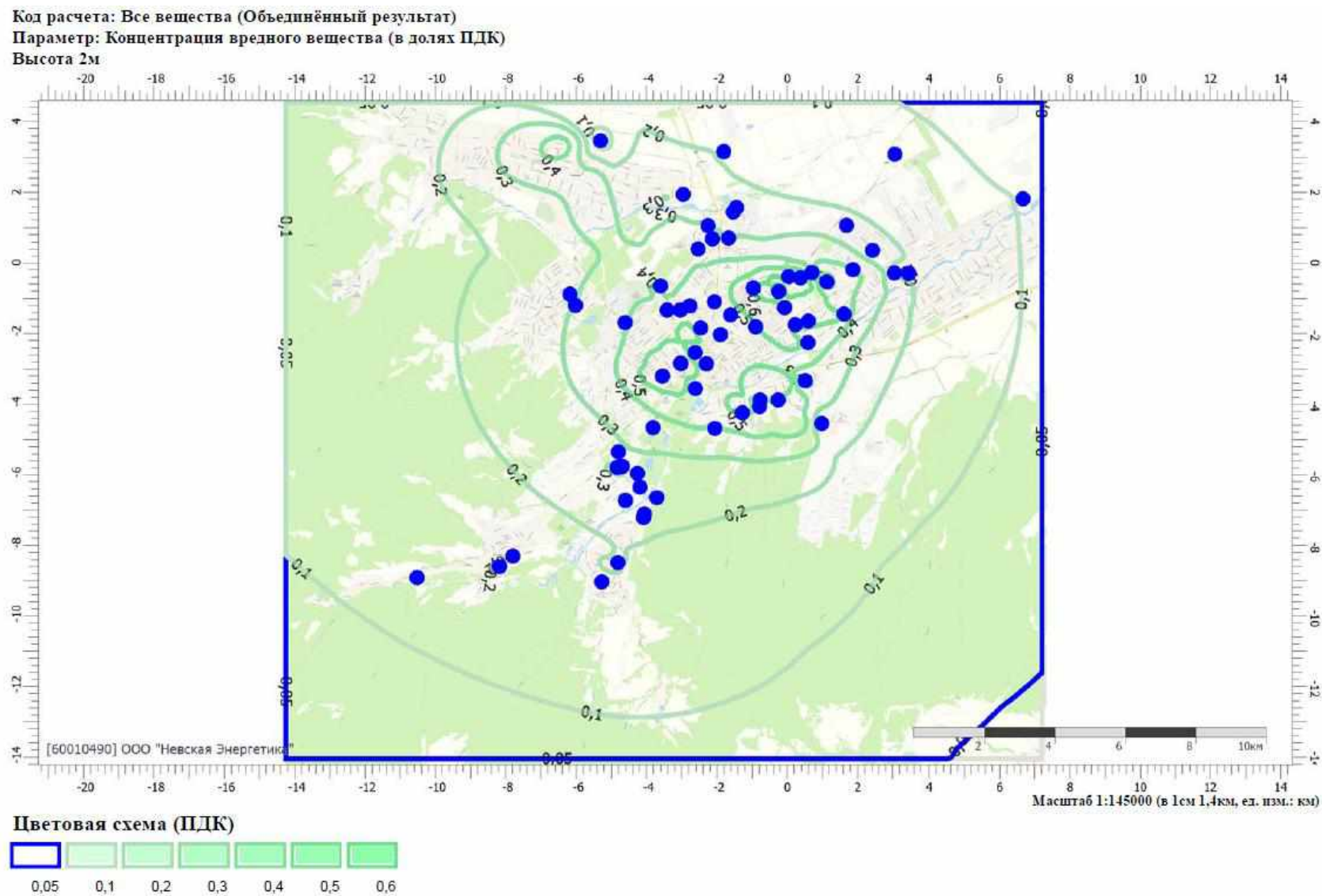
Рисунок 16.1. Среднегодовые концентрации загрязняющих веществ на территории городского округа Нальчик (объединенный результат)
