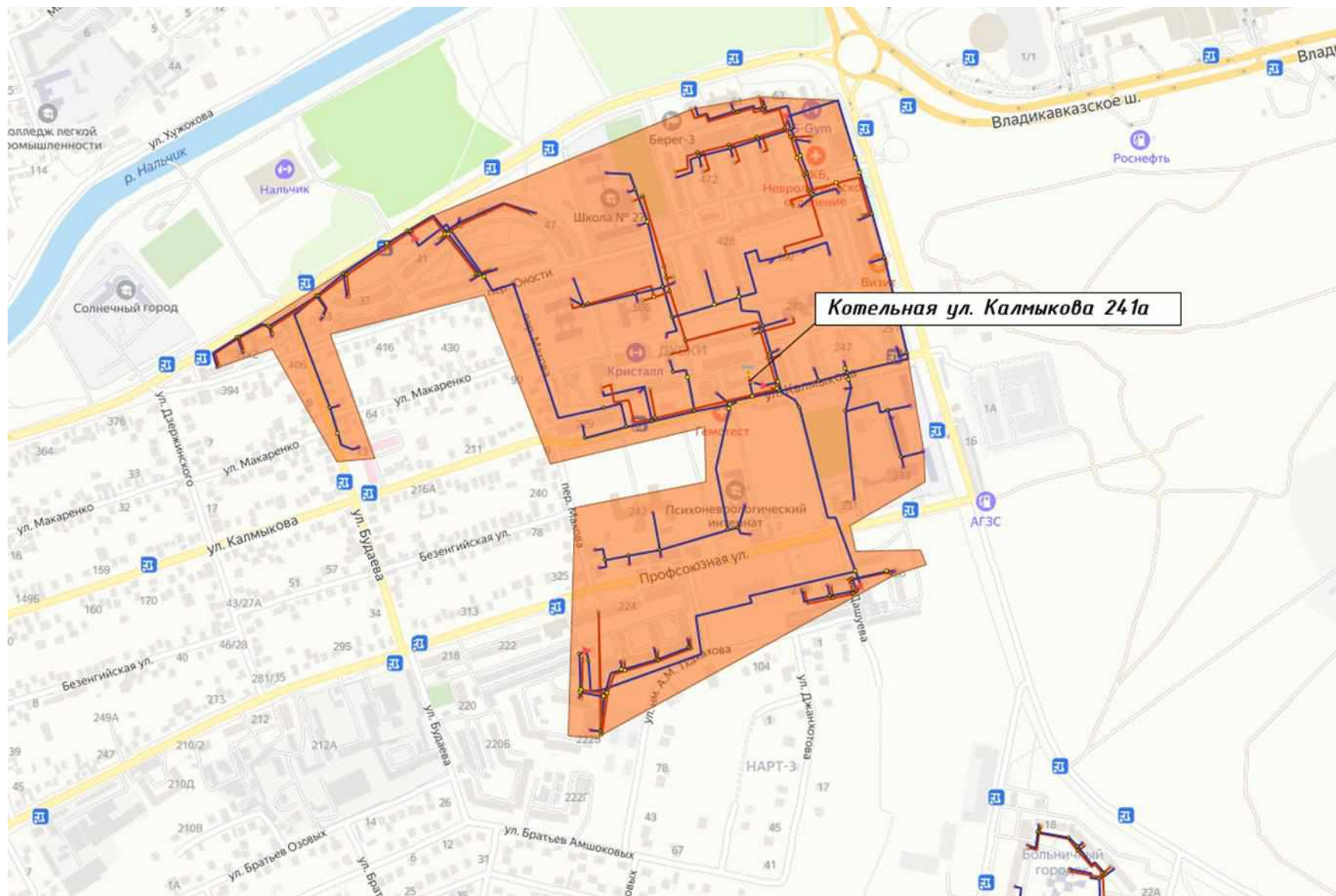
Рисунок 2.4. Существующая зона действия котельной «Калмыкова»
